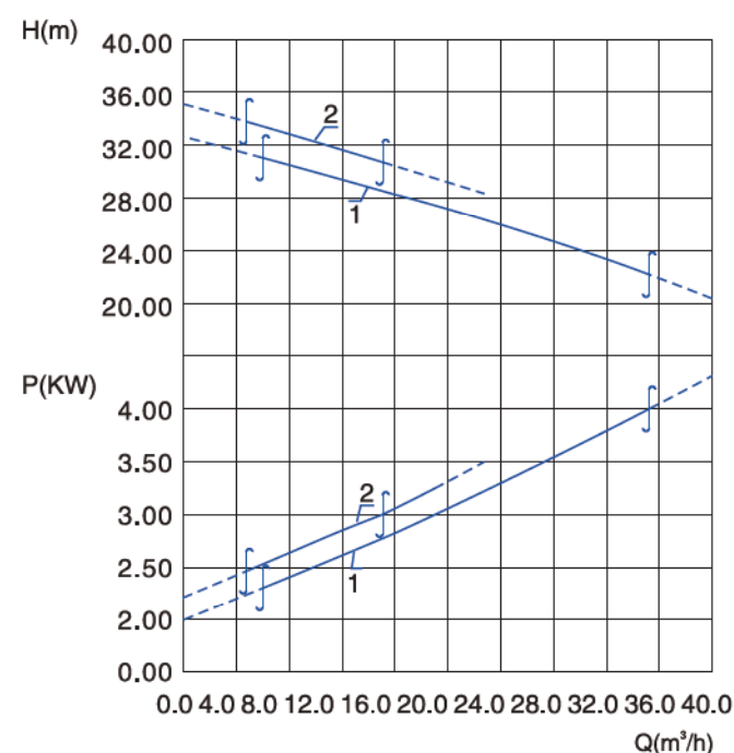
性能曲线图和主要参数例二
