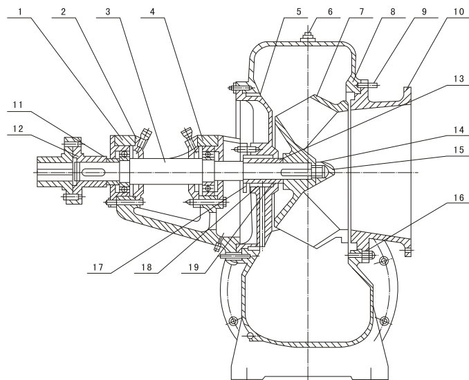
图2 400~800HW型泵结构图
